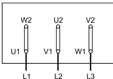
△ - Соединение 230 V (400 V)
