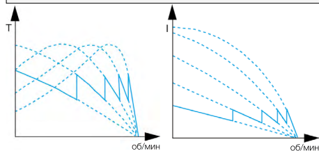
Кривая крутящего момента для двигателя с фазным ротором
