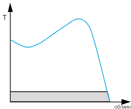
График зависимости крутящего момента от скорости при прямом пуске
