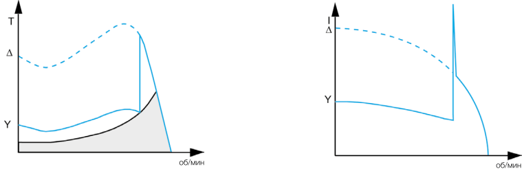
При запуске насоса могут возникнуть огромные броски тока при переключении
