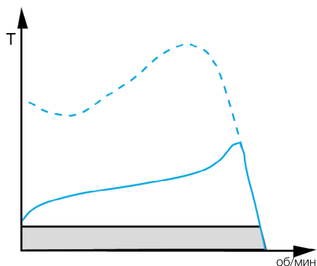
График зависимости крутящего момента от скорости при использовании устройства плавного пуска
