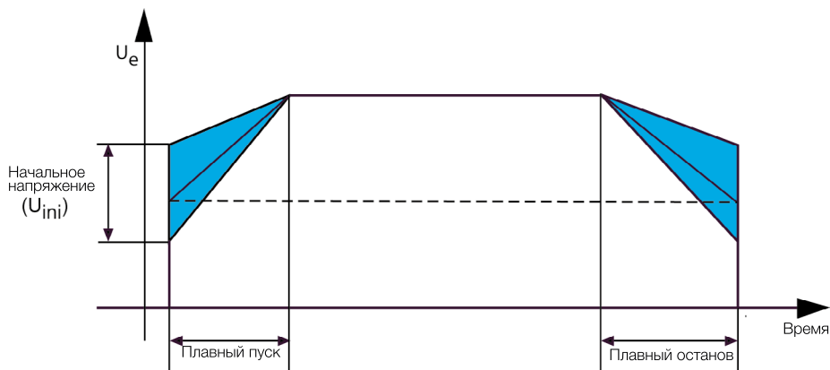
Диаграмма, на которой указано время плавного пуска, останова и начальное напряжение
