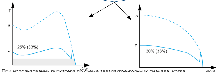
При использовании пускателя по схеме звезда/треугольник сначала, когда нагрузка невелика, ток будет снижен
