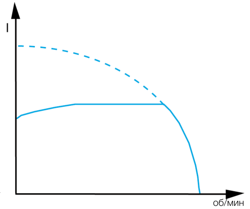
Кривые крутящего момента и тока при запуске слабо и сильно нагруженного двигателя с помощью устройства плавного пуска
