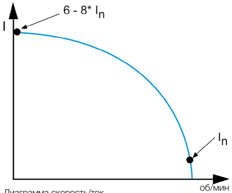
Диаграмма скорость/ток
