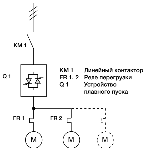
Параллельный пуск двигателей с помощью устройства плавного пуска
