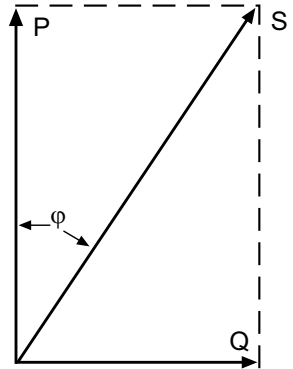
Диаграмма соотношения P , Q , S и \cos \varphi
