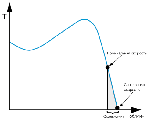
Диаграмма сравнения синхронной и номинальной скоростей
