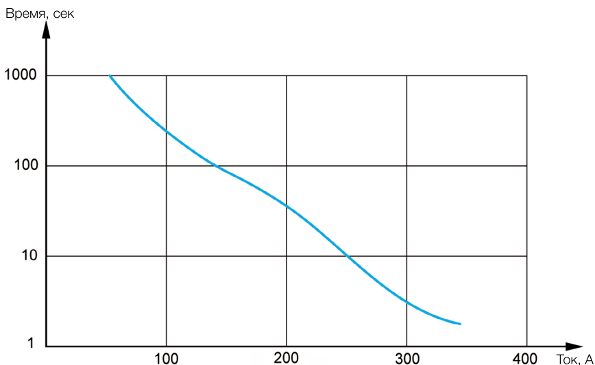
Примерный график пусковой способности для устройства плавного пуска
