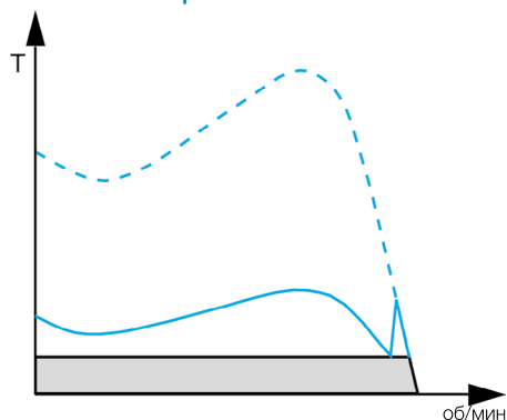
График зависимости крутящего момента от скорости при использовании пускателя со схемой соединения звезда/треугольник
