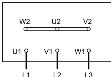
Y - Соединение 400 V (690 V)
