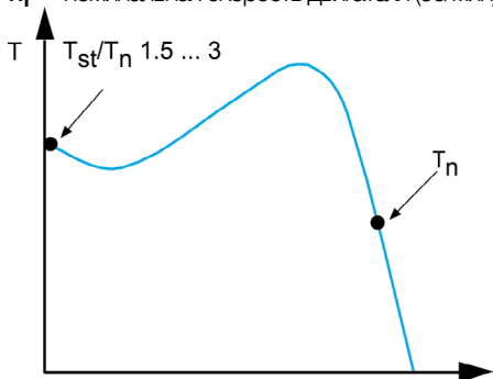
Кривая крутящего момента для двигателя с короткозамкнутым ротором
