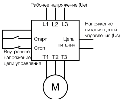
Устройства плавного пуска с внутренним напряжением цепи управления
