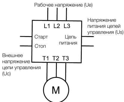
Устройства плавного пуска с внешним напряжением цепи управления
