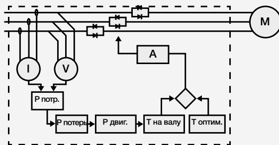
Алгоритм управления крутящим моментом
