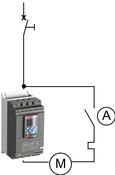
Вариант А Главный контактор находится внутри треугольника
