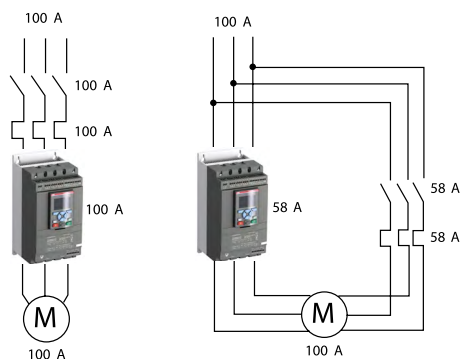
Устройство плавного пуска при подключении в линию
