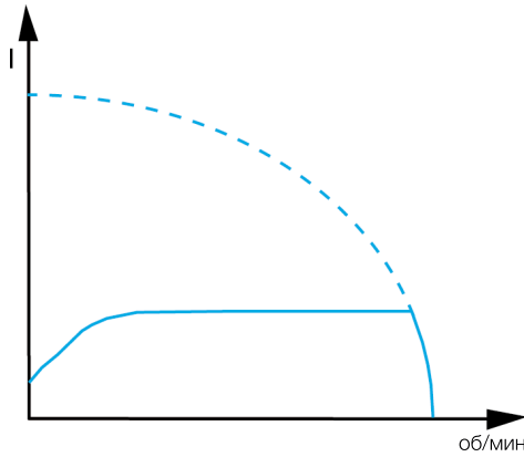
Кривые крутящего момента и тока при запуске слабо и сильно нагруженного двигателя с помощью устройства плавного пуска
