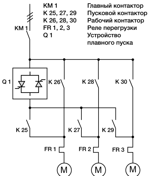
Последовательный пуск двигателей с помощью устройства плавного пуска
