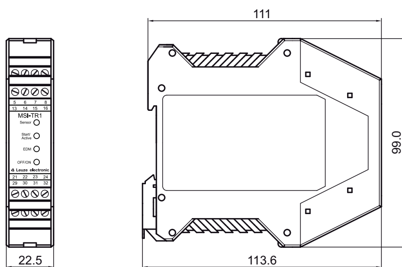
Рис. 14.1: Размеры MSI-TR1
