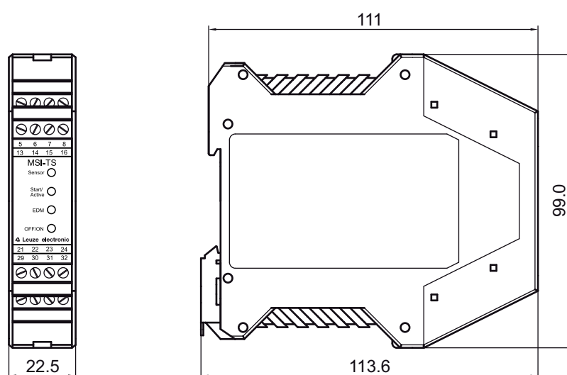
Рис. 14.3: Размеры MSI-TS
