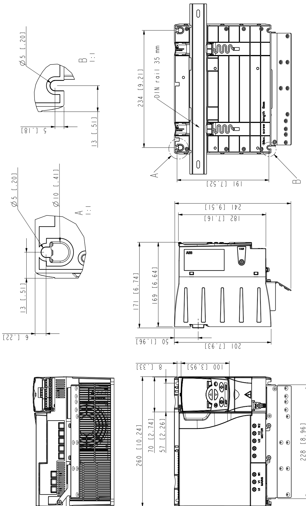
Типоразмер R4, IP20 (монтаж в шкафу) / UL, открытое исполнение
